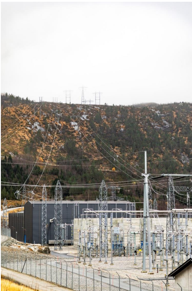
Die NordLink Konverterstation in Tonstad, Außenaufnahme vom November 2020. Im Vordergrund die Schaltfelder.
